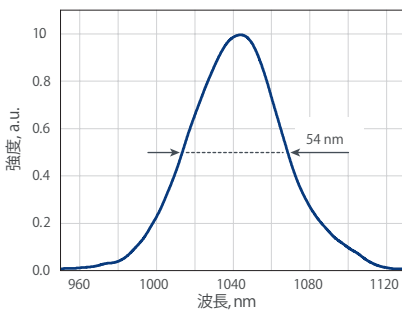
FLINT-FL2-SPのスペクトル（典型値）
